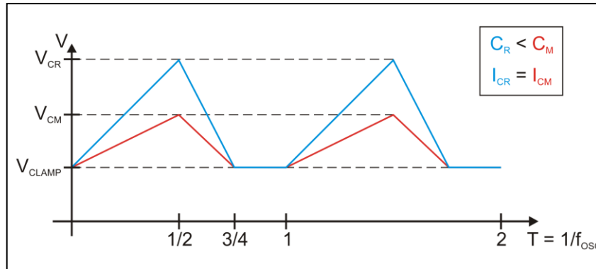
图 4: 二个积分器的电压输出
