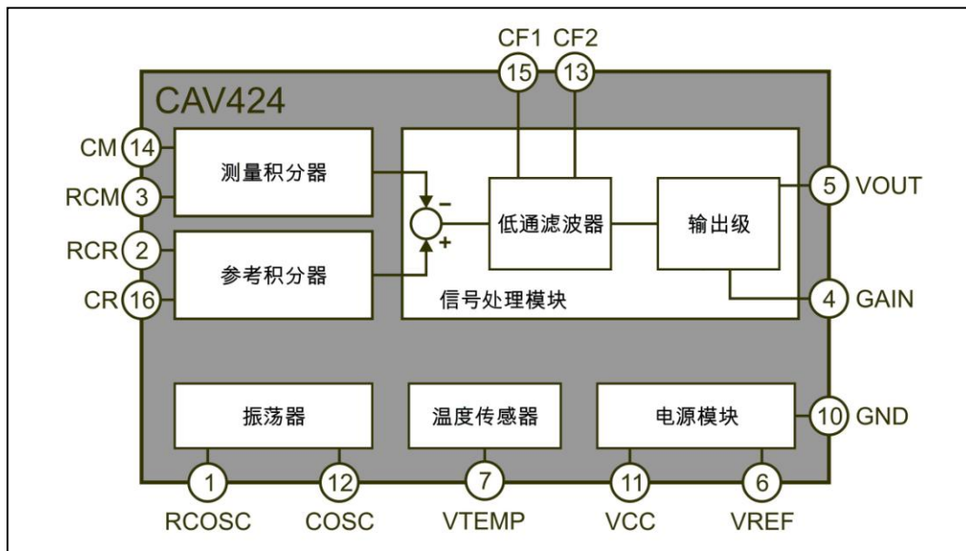
图 1 : CAV424 电路方框图
