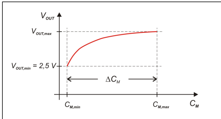
图 5: 输出电压信号 V_{OUT} 与测量电容 C_M 的关系
